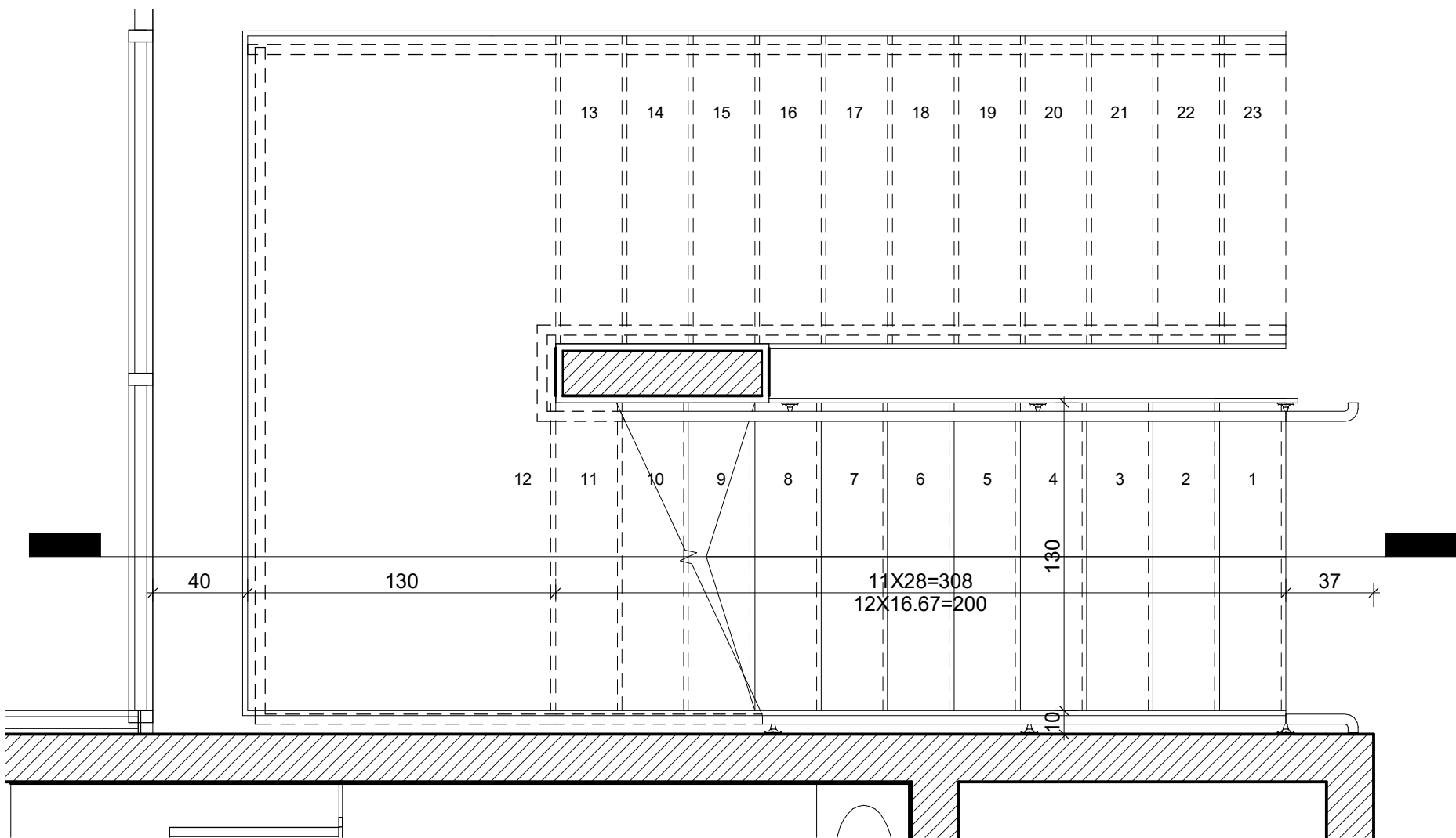
תכנית מדרגות כניסה- קומת קרקע 1 : 25
