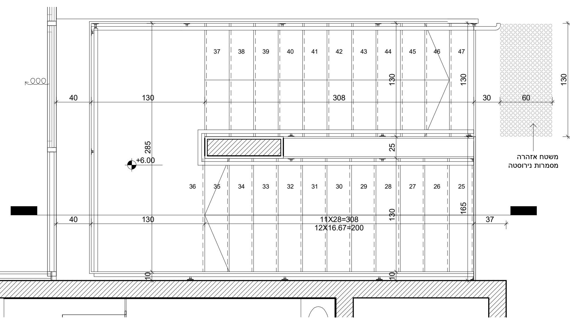
תכנית מדרגות כניסה- קומה ב 1 : 25
