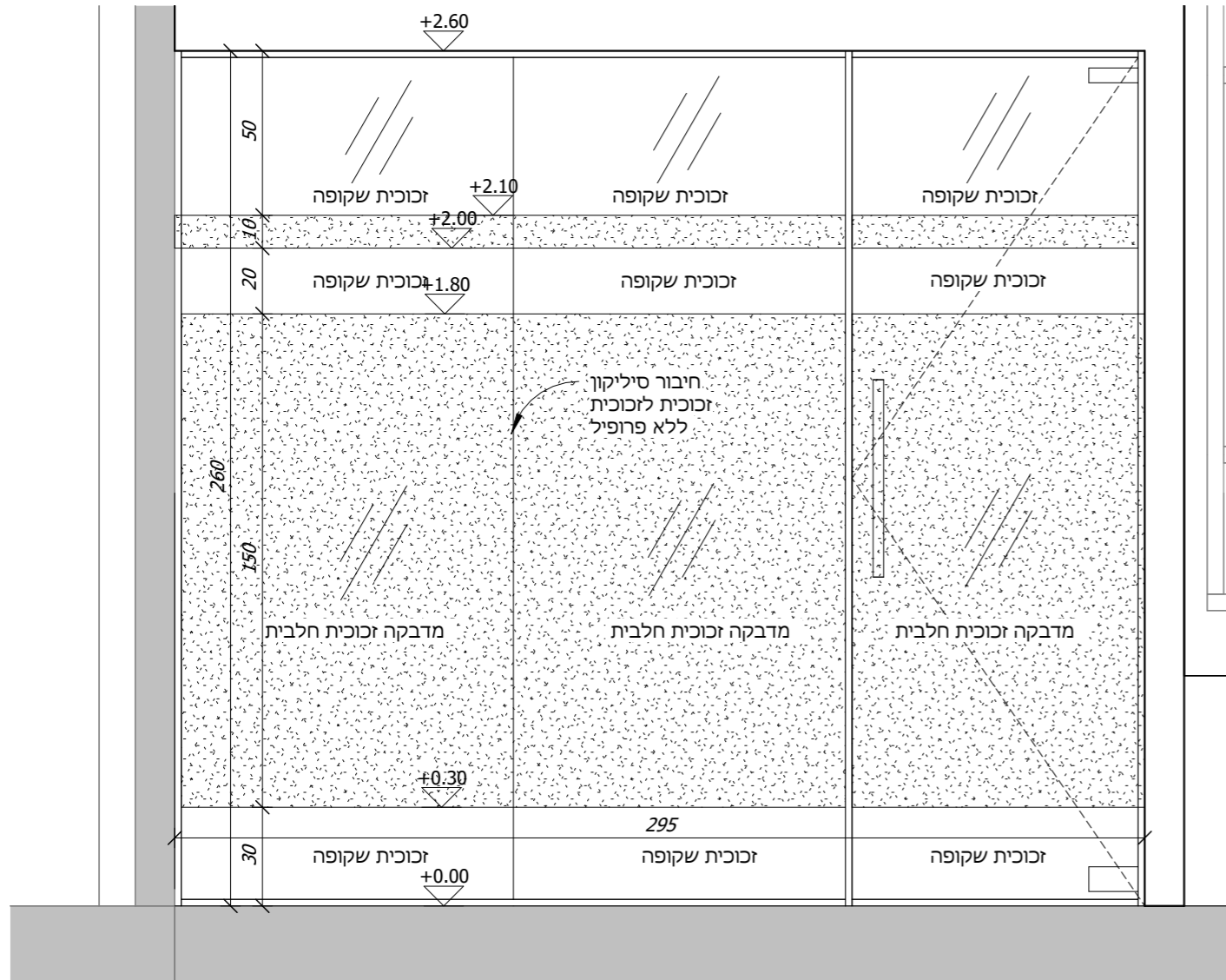
חזית א-05 1 : 20
