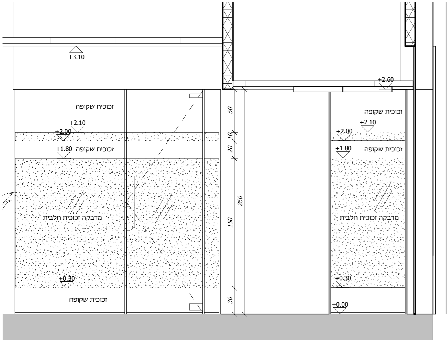
חזית-א-04
