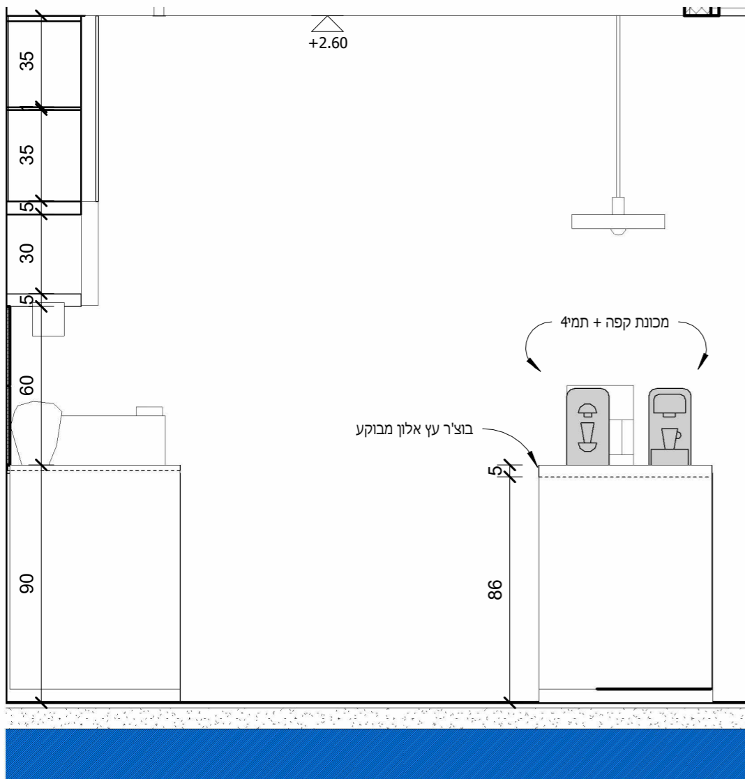
חזית 1 מטבחון
