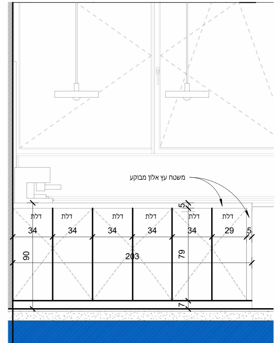
חתך 1 מטבחון
