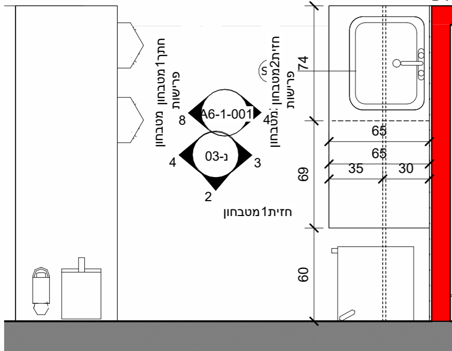
חזית 1 מטבחון
