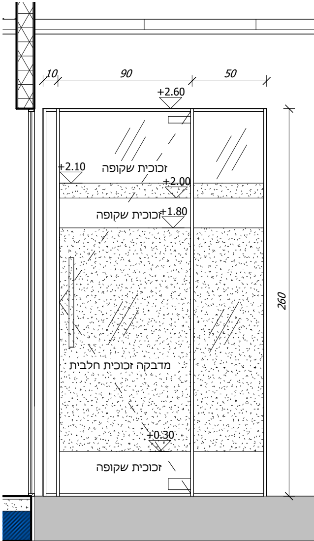
חזית א-07
