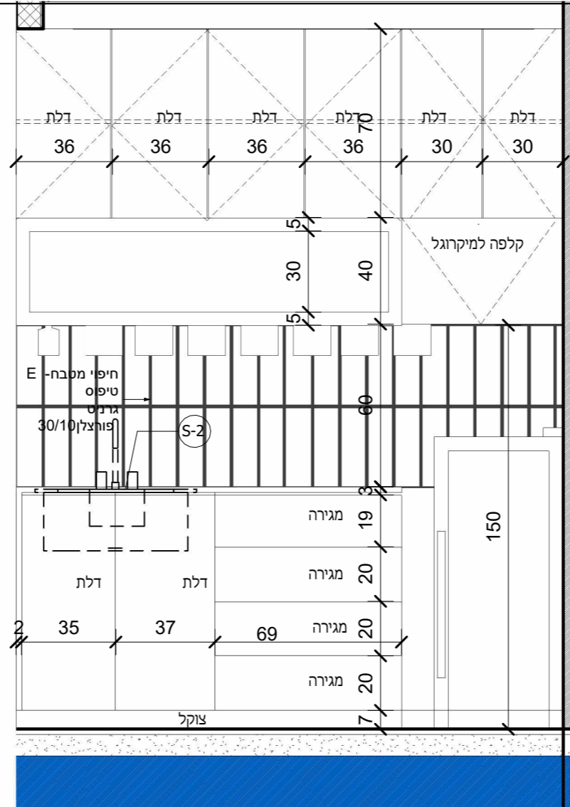
חזית 2 מטבחון
