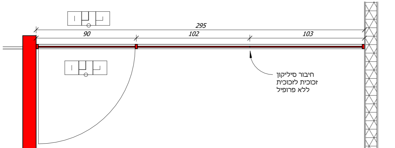
חזית א-05 1 : 20
