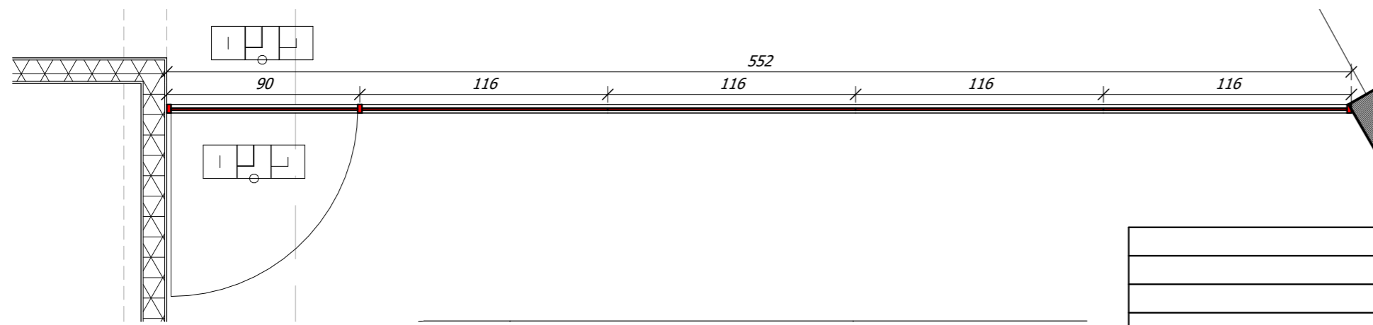
תכנית א-06 1 : 25
