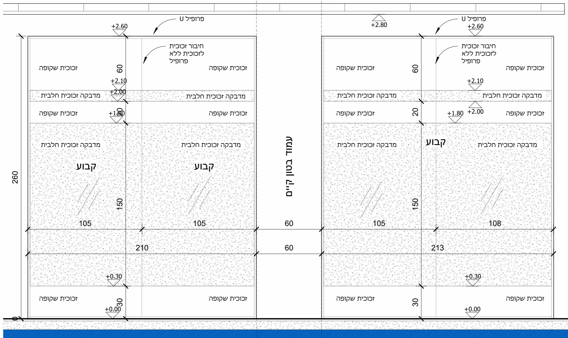
חזית-א-02 1 : 20
